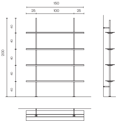
EXAMPLE 1 Dimensions 150 x 25 x 200 cm 59 x 9,8 x 78,7 "
