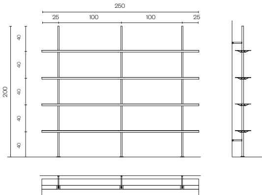
EXAMPLE 3 Dimensions 250 x 25 x 200 cm 98,4 x 9,8 x 78,7 "
