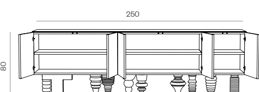
Module: 1B + 1B + 3B
