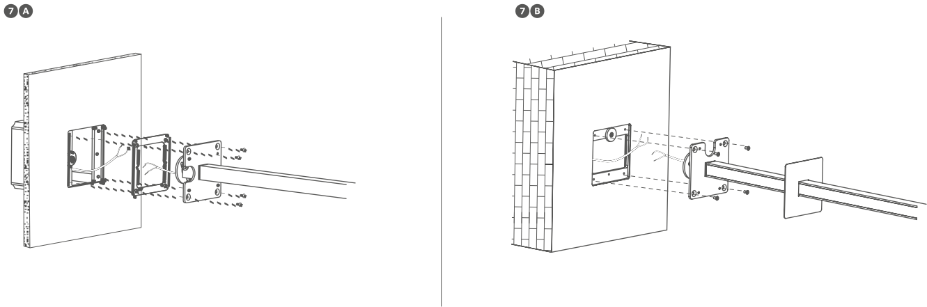
Setting for the perpendicularity of the lamp to the wall / Regolazione per la perpendicolarità della lampada al muro
