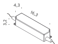
60W / LIN ALI 31
